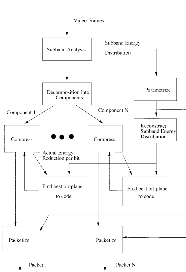
Fig. 5. Encoding procedures.
